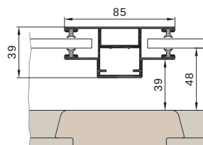
Kämpfer mit freitragender Führungsschiene
